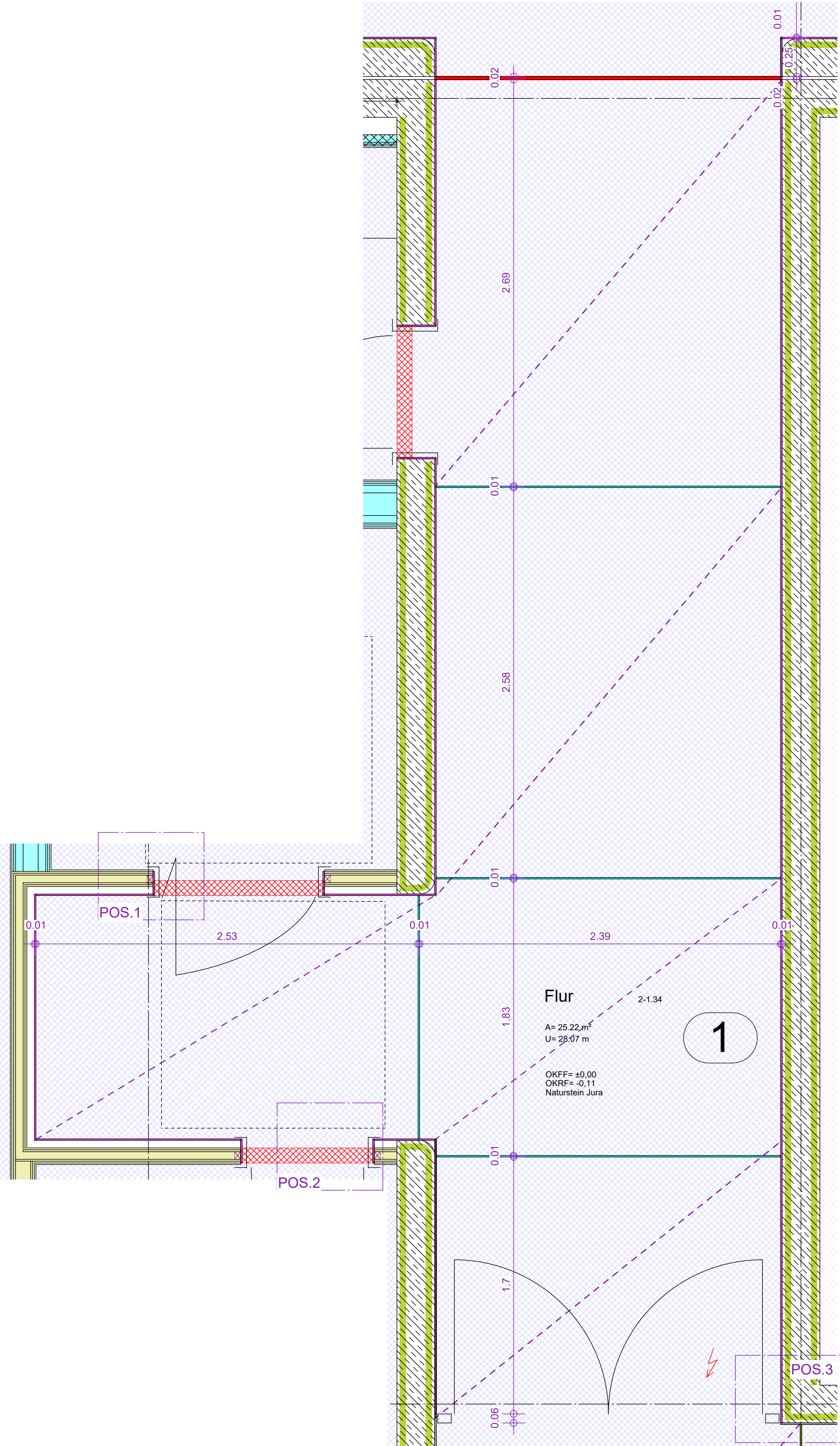
EG GRUNDRISSAUSSCHNITT ESTRICHARBEITEN Flur 2-1.34 M 1:20
